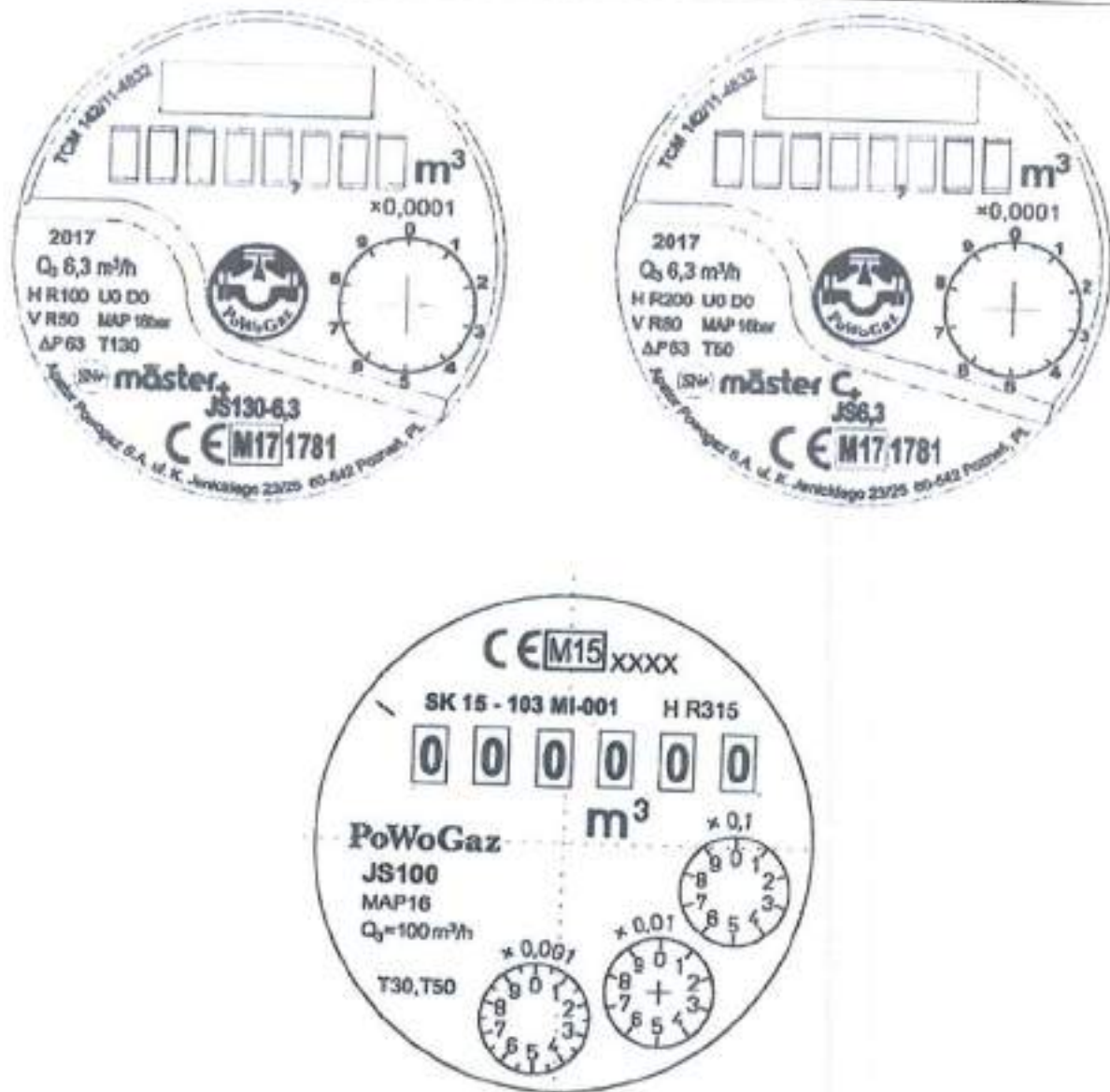
Рисунок 12 – Маркування лічильника
